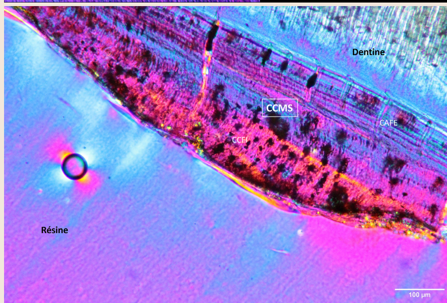
Section de quatrième prémolaire inférieure (P4) de cerf ( Cervus elaphus ). Observation microscopique en lumière transmise polarisée et avec lame d'onde ( \lambda ), x100. CAFE : ciment acellulaire à fibres extrinsèques ; CCFI : ciment cellulaire à fibres intrinsèques ; CCMS : ciment cellulaire mixte stratifié ; CH : couche hyaline ; CGT : couche granuleuse de Tomes.
